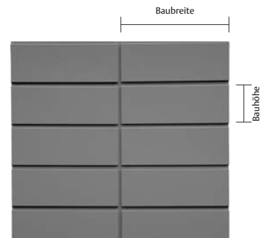
Fassadeneinteilung mit mittigen und oberen Pass - Kassetten
